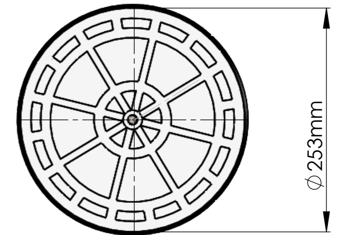
VISTA INFERIOR
