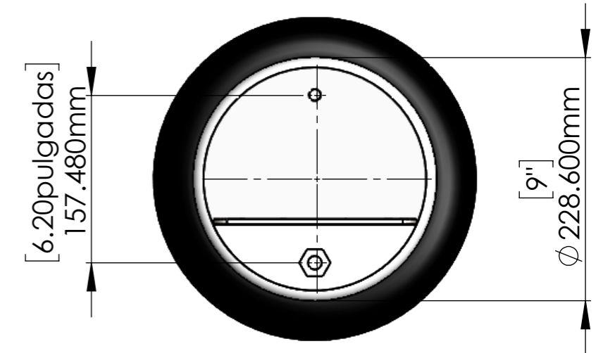
VISTA SUPERIOR
